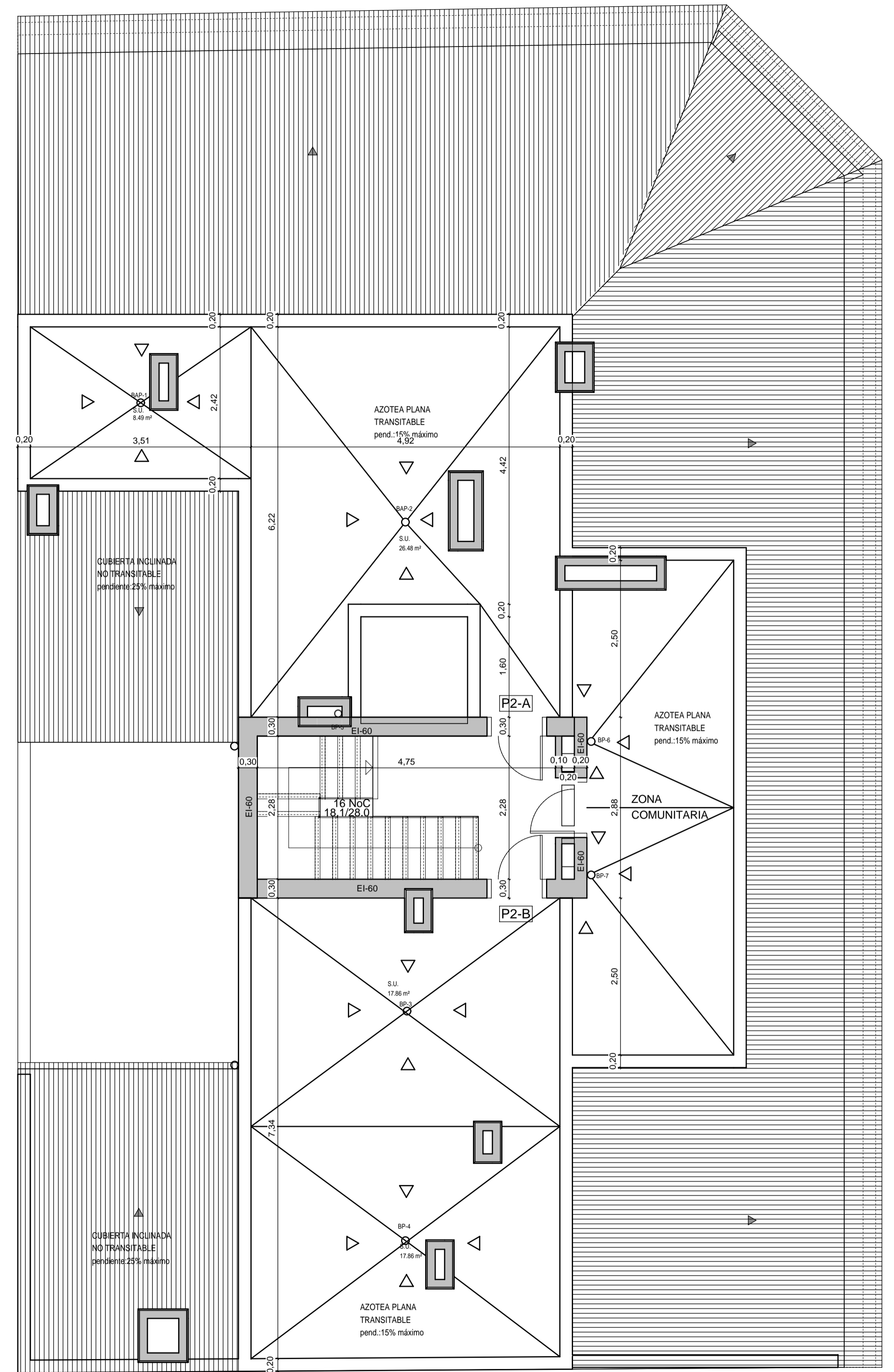
PLANTA CUBIERTA
