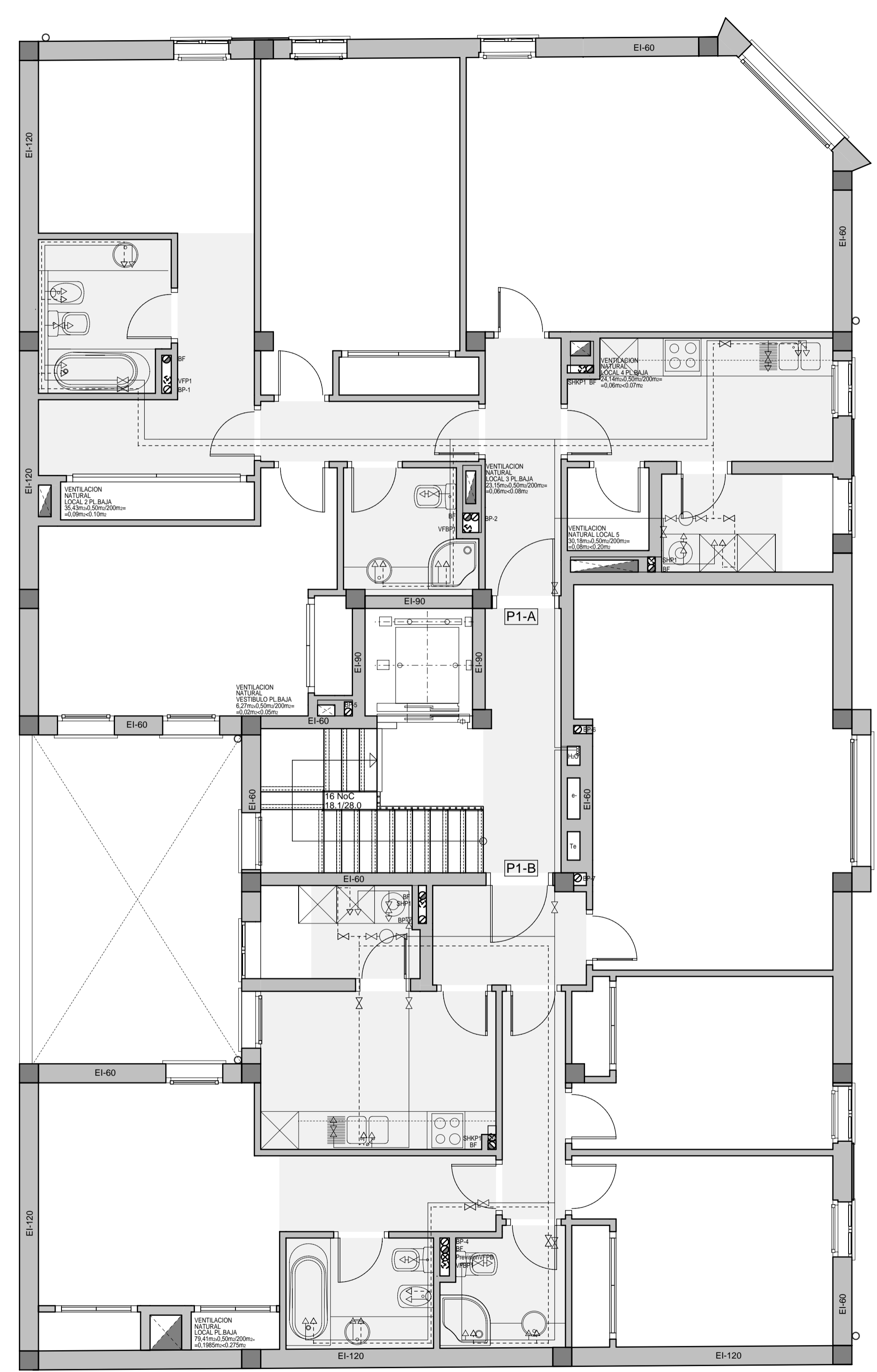
PLANTA PISO 1º
