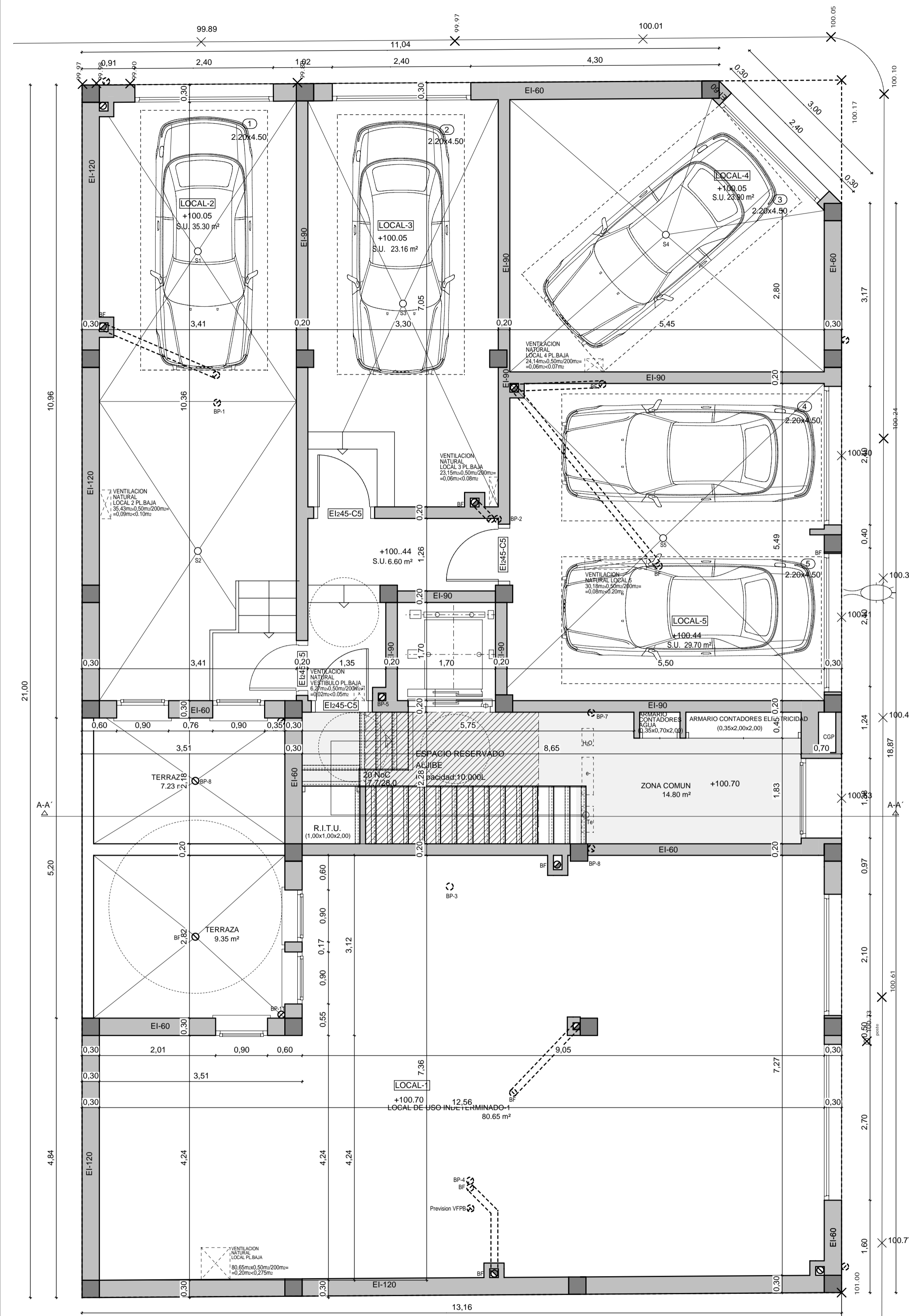
PLANTA BAJA
