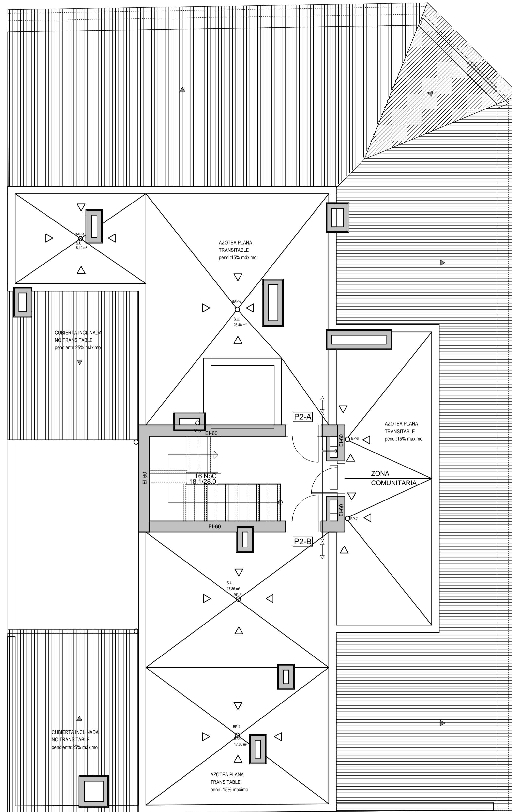
PLANTA CUBIERTA
